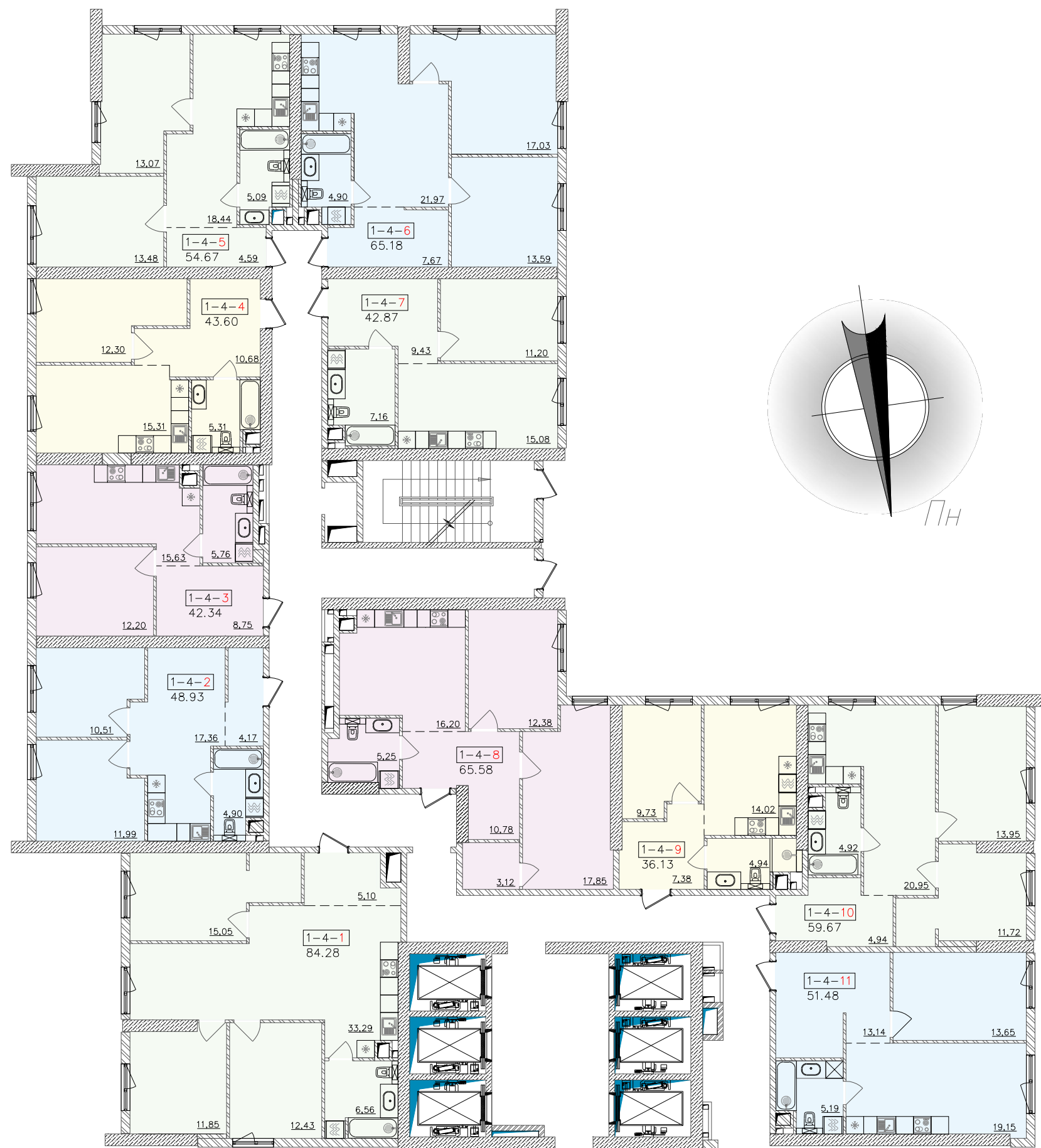
ПЛАН 4 ПОВЕРХУ ЖК "64 Перлина" 1 секція
