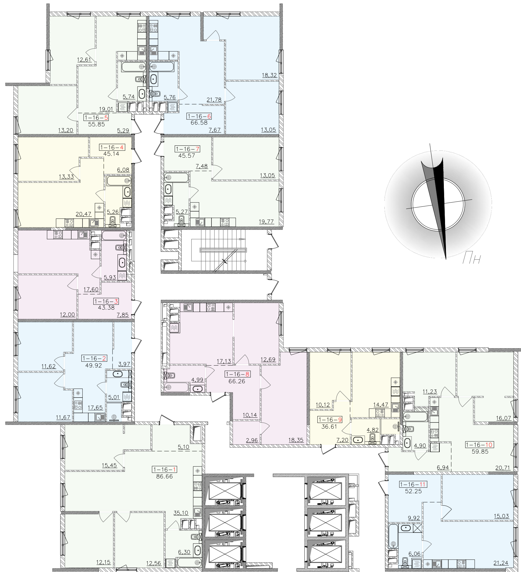
ПЛАН 16 ПОВЕРХУ ЖК "64 Перлина" 1 секція
