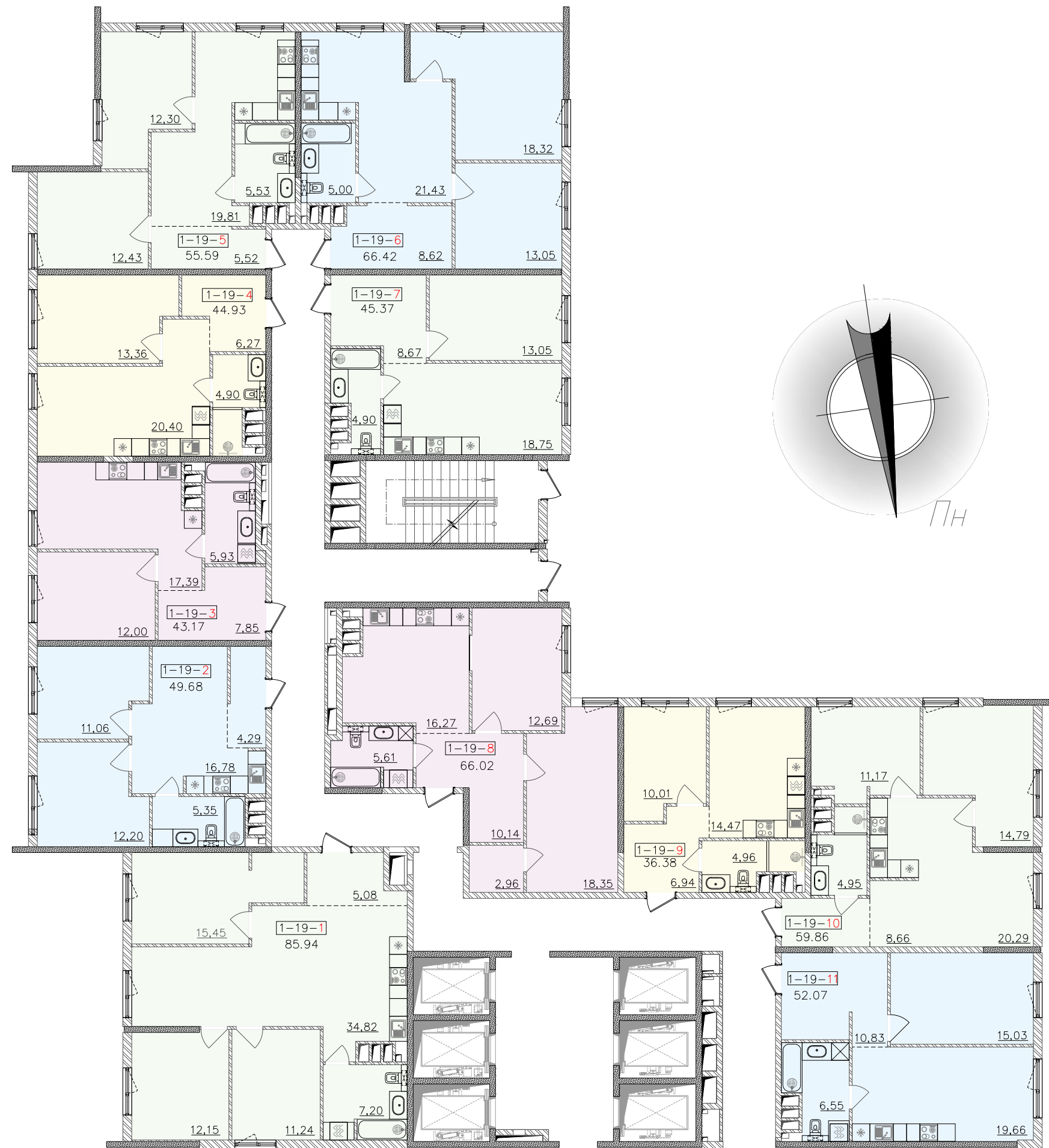
ПЛАН 19 ПОВЕРХУ ЖК "64 Перлина" 1 секція
