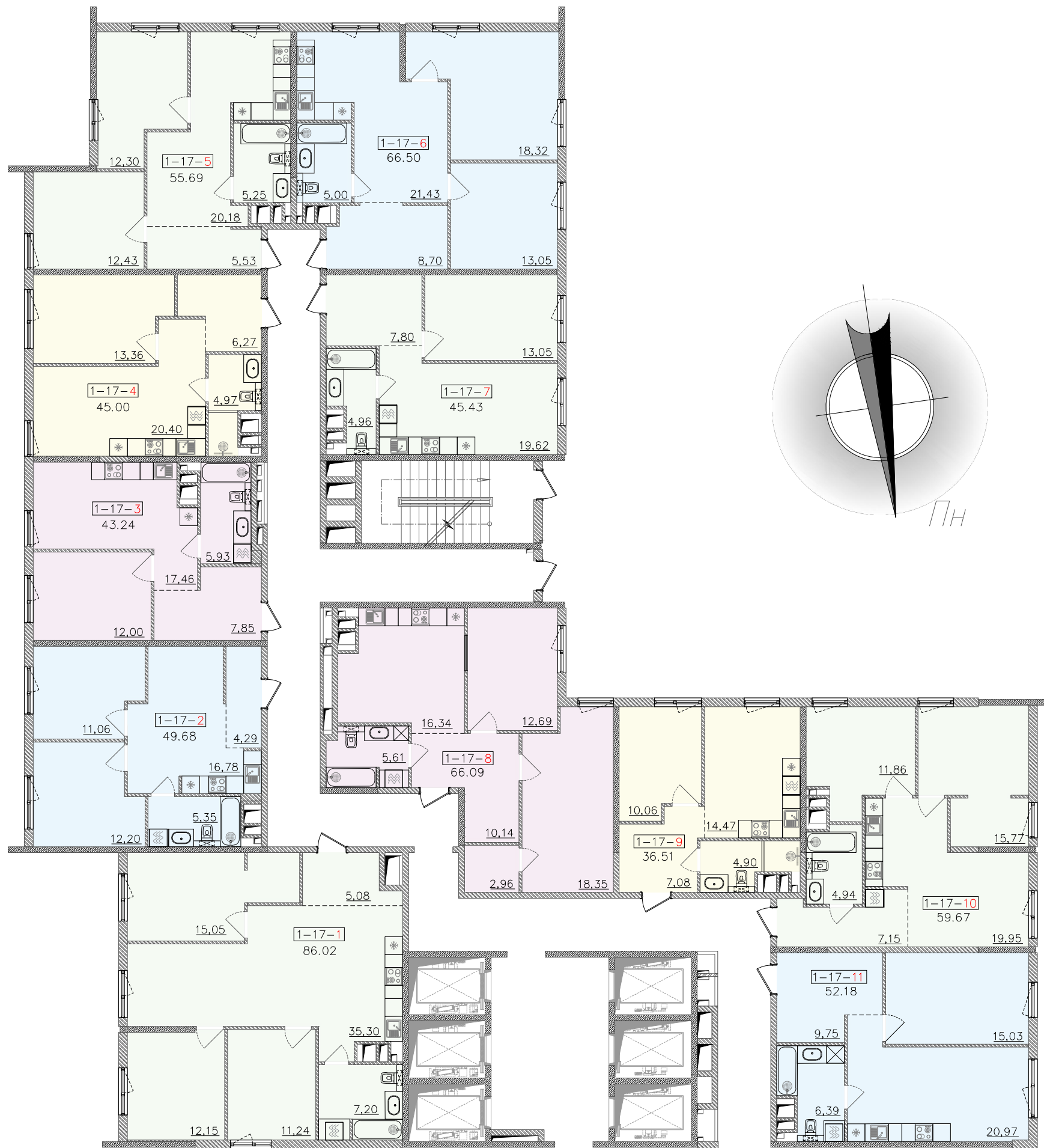
ПЛАН 17 ПОВЕРХУ ЖК "64 Перлина" 1 секція
