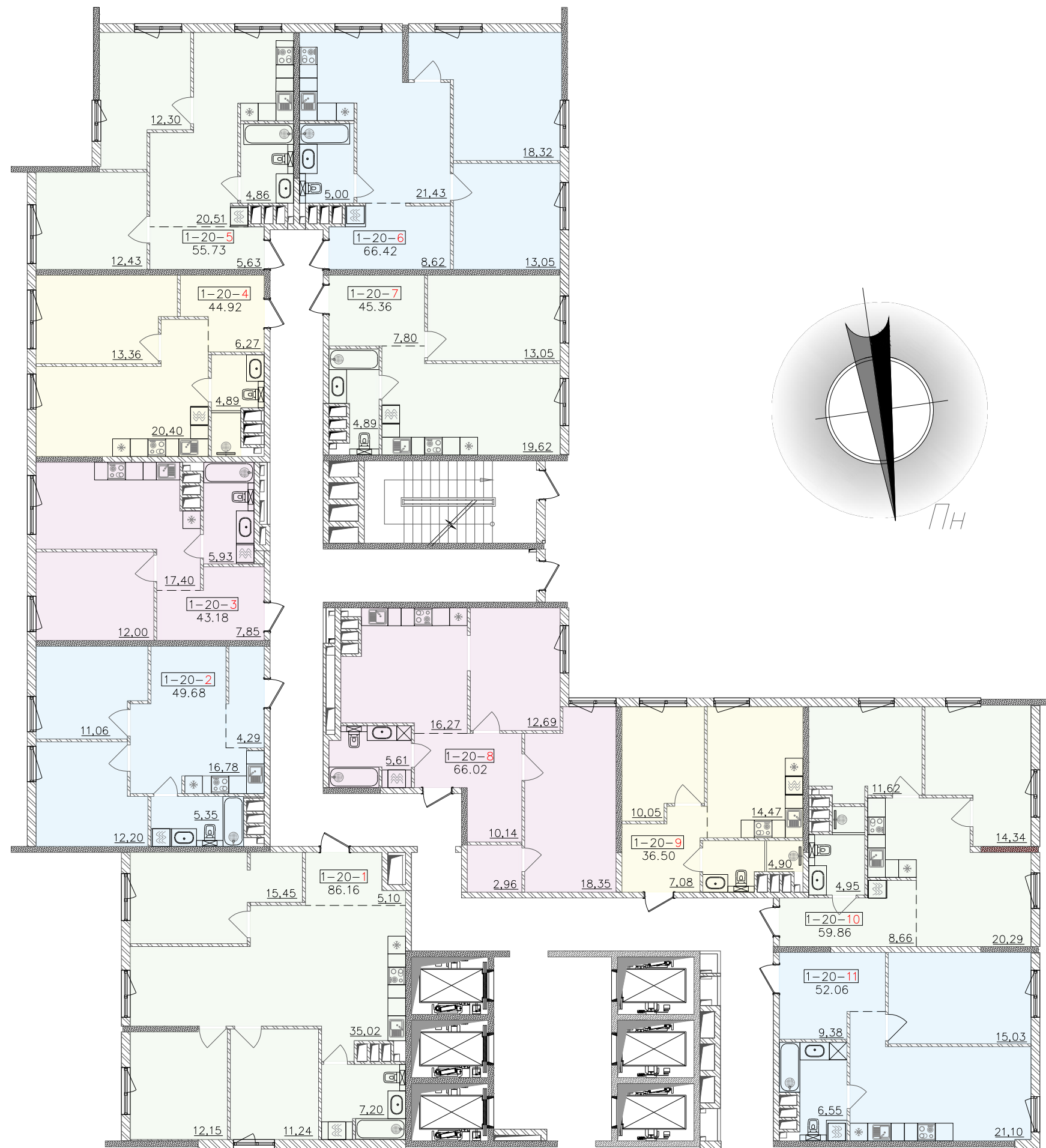
ПЛАН 20 ПОВЕРХУ ЖК "64 Перлина" 1 секція
