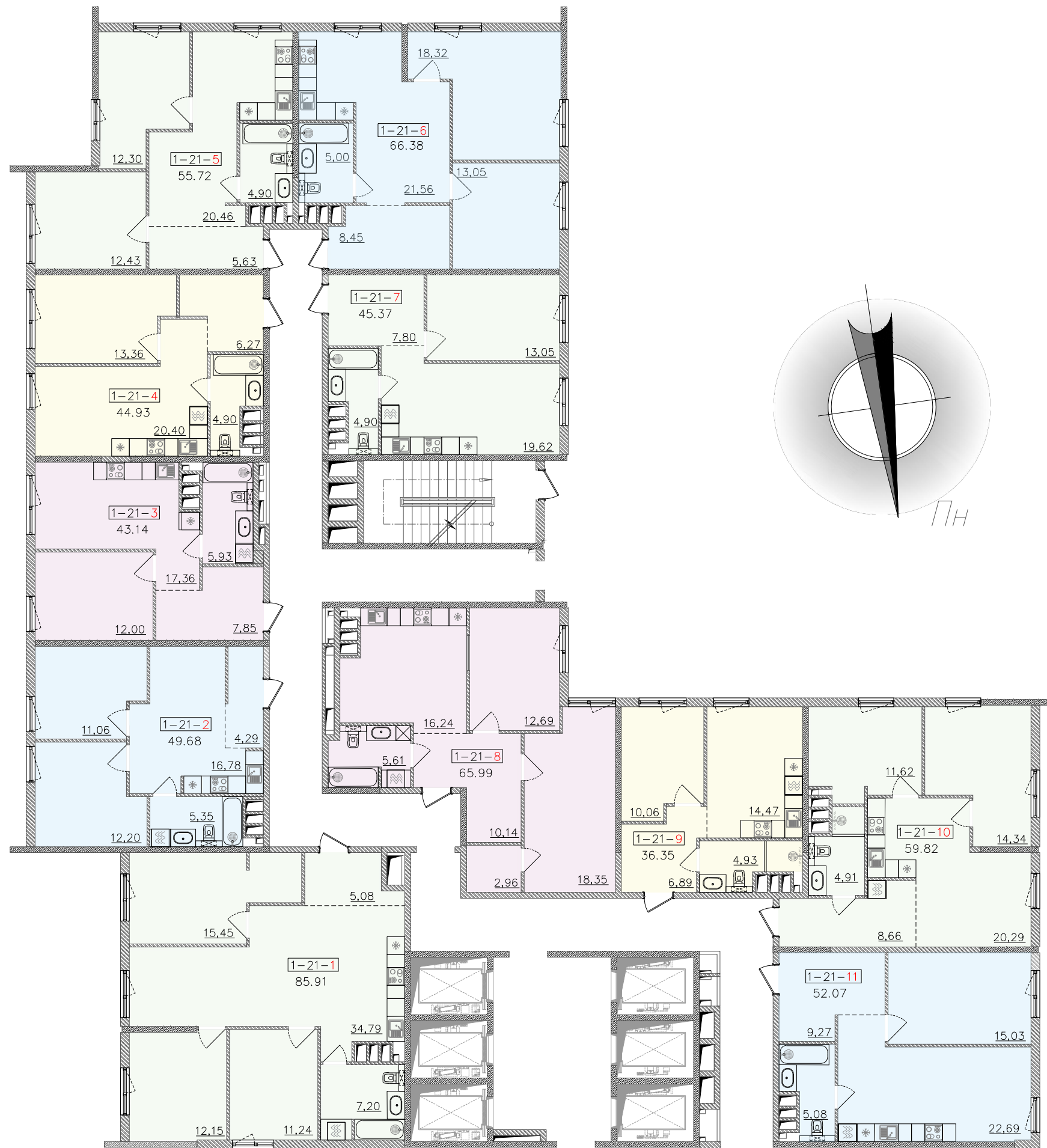
ПЛАН 21 ПОВЕРХУ ЖК "64 Перлина" 1 секція
